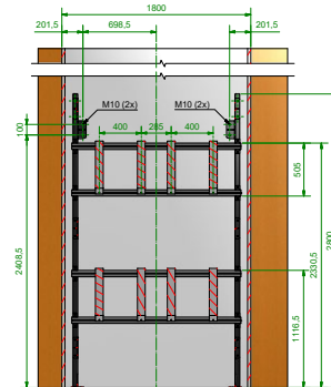
B-B 1:20
